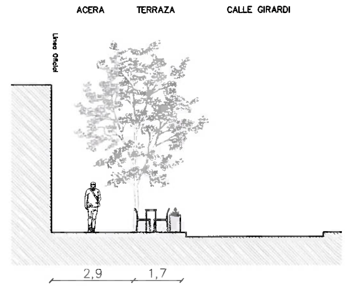
CORTE A-A'
