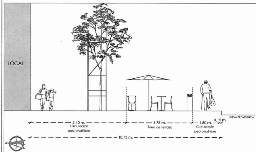
CORTE A-A'
