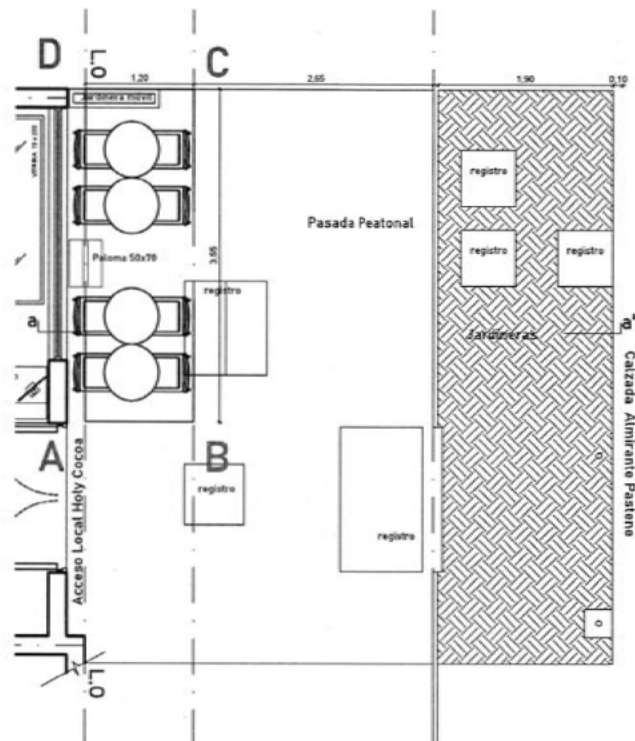
Planta terraza, escala 1:50
