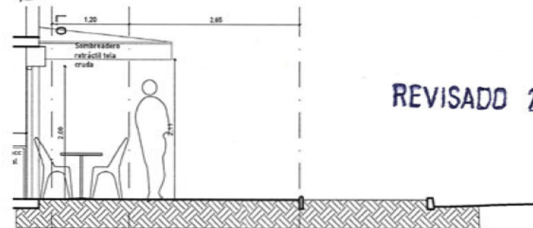
Corte a-a' escala 1:50
