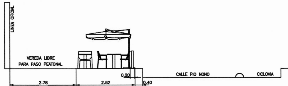
CORTE A-A ESC: 1/60
