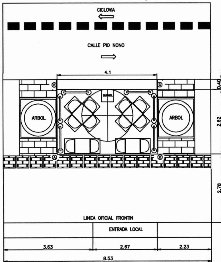
VISTA EN PLANTA ESC: 1/60
