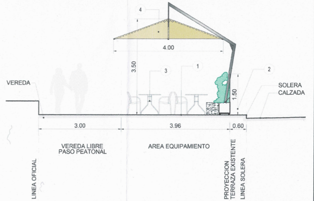
SECCION 1
