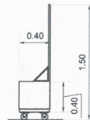
ELEV. LAT.
