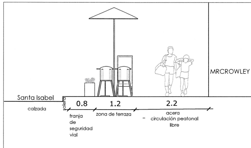
CORTE A-A'
