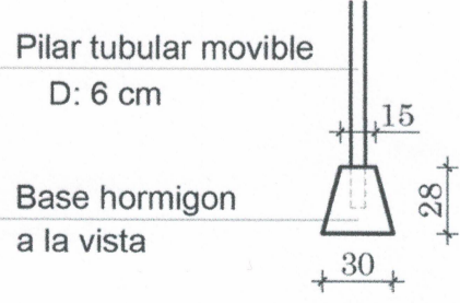
Elevacion Base Hormigon Movil
