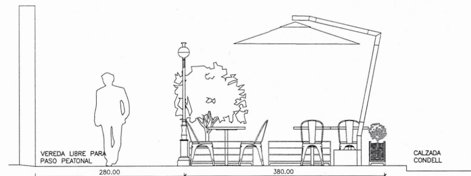
CORTE A-A
