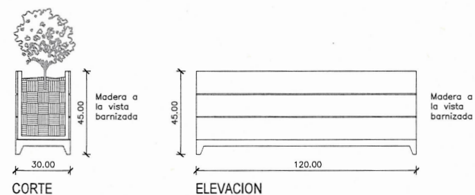
DETALLE DE JARDINERA
