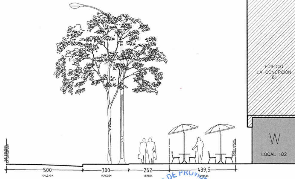
CORTE 1-1 ESC 1/100
