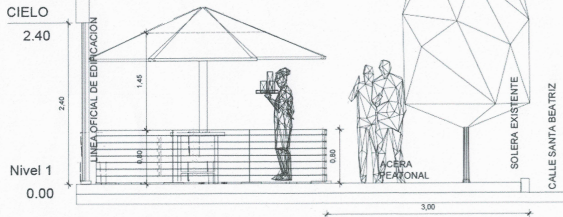
CORTE A-A
