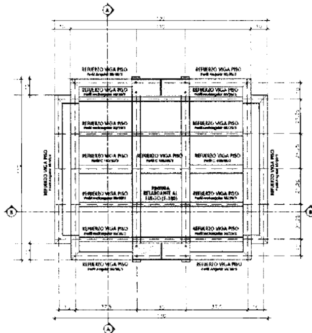
PLANTA ESQUEMATICA REFUERZO ESTRUCTURAL PISO ASCENSOR
