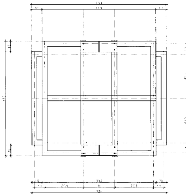
PLANTA ESQUEMATICA SITUACIÓN ACTUAL PISO ASCENSOR
