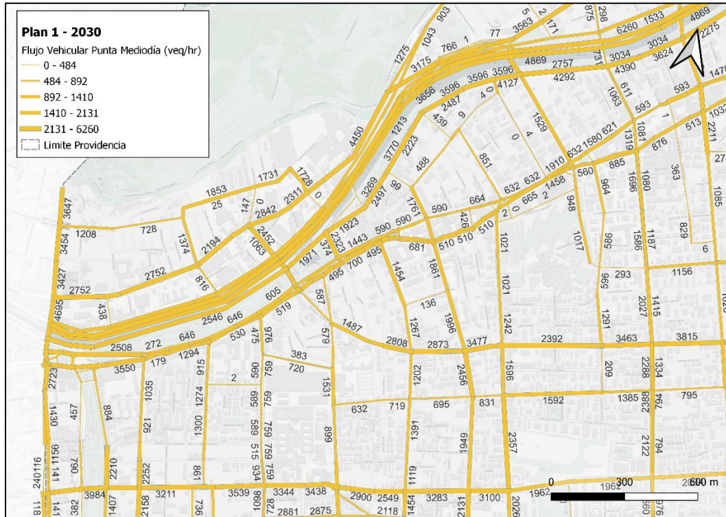
FIGURA Nº 4.8-53: FLUJO TOTAL SECTOR NORPONIENTE – PLAN 1 2030 PUNTA MEDIODÍA
