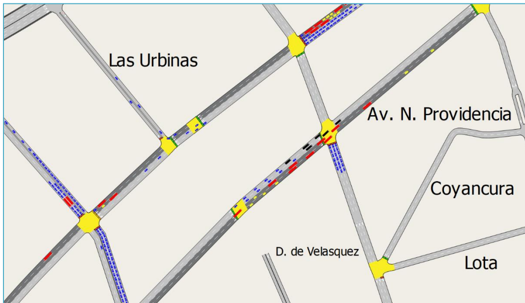
FIGURA N° 5.2-63: MICROSIMULACIÓN PLAN DE PROYECTOS CALLE PEATONAL GUARDIA VIEJA Y DIEGO DE VELÁSQUEZ
