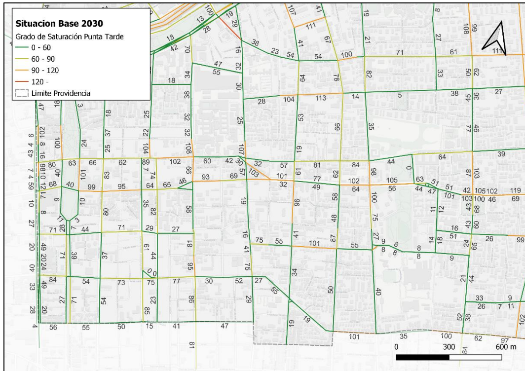
FIGURA Nº 4.8-32: GRADO DE SATURACIÓN SECTOR SURPONIENTE– SITUACIÓN BASE 2030 PUNTA TARDE
