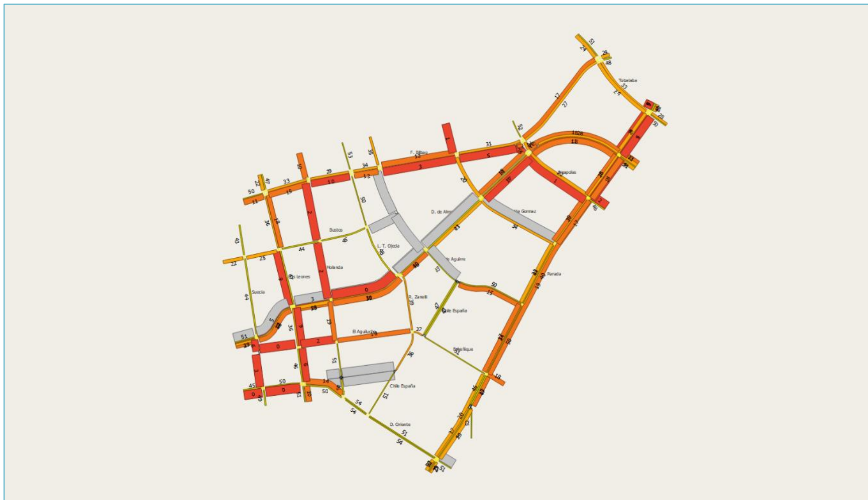
FIGURA N° 5.2-99: VELOCIDAD SIMULADA ÁREA DE MICROSIMULACIÓN 2 PLAN DE PROYECTOS PUNTA TARDE
