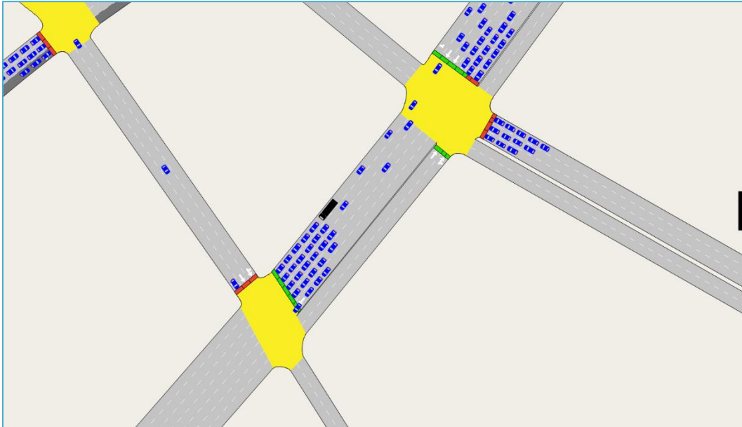
FIGURA N° 5.2-54: MICROSIMULACIÓN SITUACIÓN BASE FIN REVERSIBILIDAD Y REDISEÑO ANDRÉS BELLO
