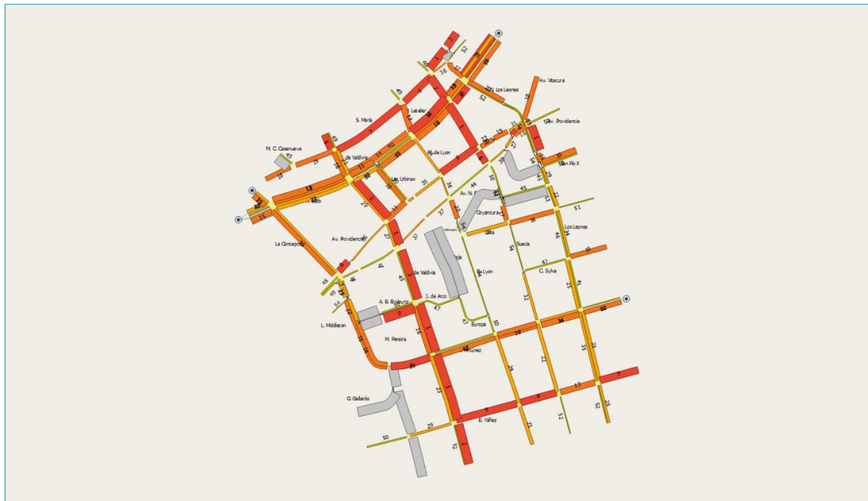
FIGURA N° 5.2-67: VELOCIDAD SIMULADA ÁREA DE MICROSIMULACIÓN 1 PLAN DE PROYECTOS PUNTA MAÑANA
