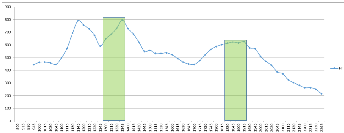
FIGURA Nº 2.3-30: FLUJO TOTAL PARA CICLOS (FTI) SÁBADO, HORA REPRESENTATIVA POR PERÍODO
