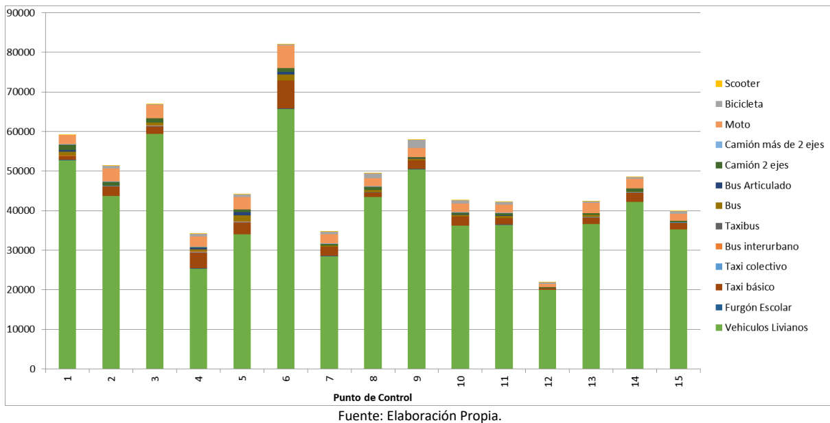
FIGURA Nº 2.3-21: FLUJO TOTAL MEDIDO POR PUNTO DE CONTROL - DÍA LABORAL
