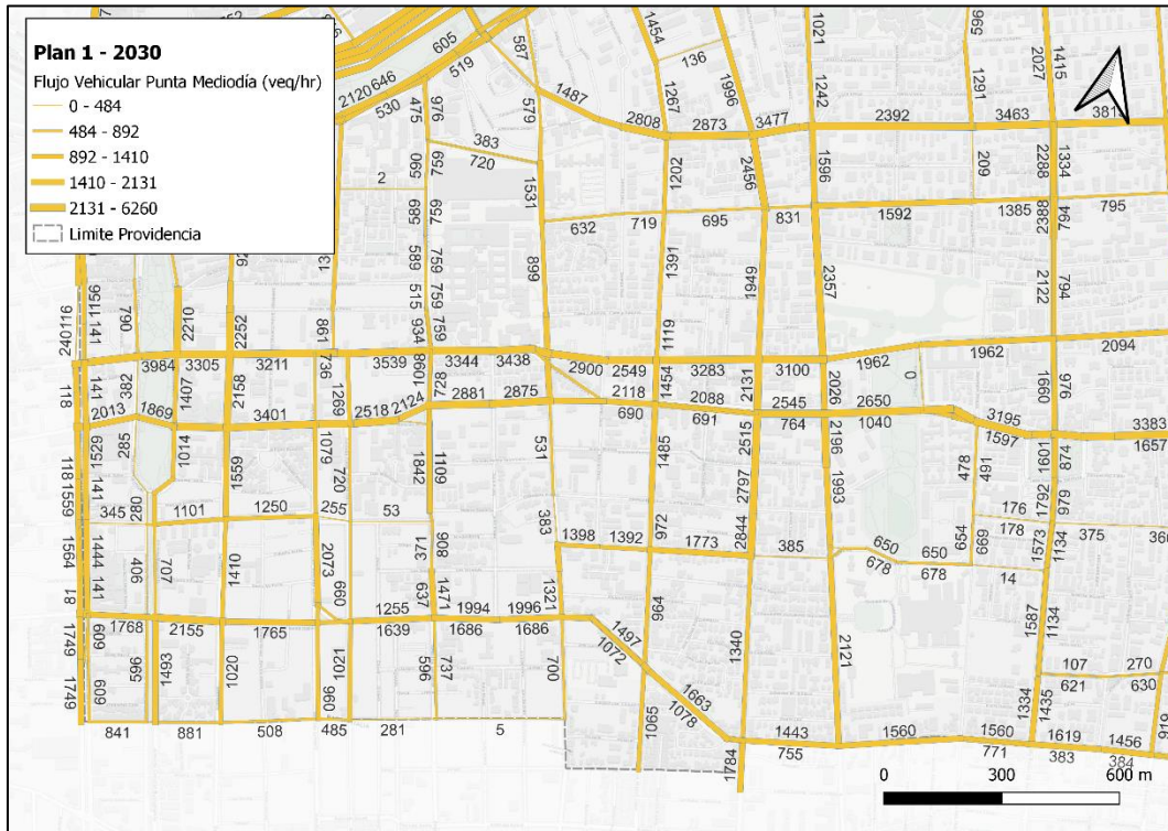
FIGURA Nº 4.8-55: FLUJO TOTAL SECTOR SURPONIENTE – PLAN 1 2030 PUNTA MEDIODÍA
