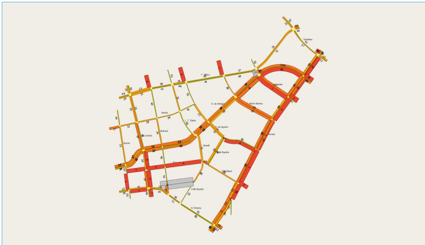
FIGURA N° 5.2-97: VELOCIDAD SIMULADA ÁREA DE MICROSIMULACIÓN 2 PLAN DE PROYECTOS FUERA DE PUNTA
