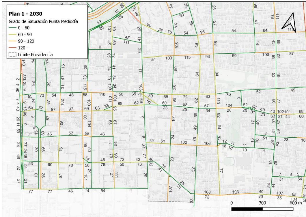
FIGURA Nº 4.8-56: GRADO DE SATURACIÓN SECTOR SURPONIENTE– PLAN 1 2030 PUNTA MEDIODÍA
