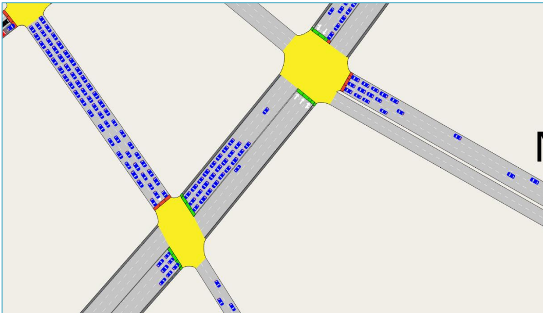
FIGURA N° 5.2-55: MICROSIMULACIÓN PLAN DE PROYECTOS FIN REVERSIBILIDAD Y REDISEÑO ANDRÉS BELLO
