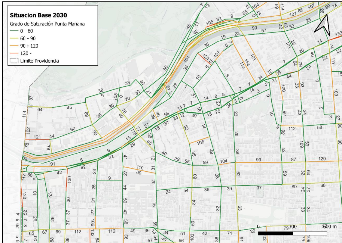
FIGURA Nº 4.8-6: GRADO DE SATURACIÓN SECTOR NORPONIENTE-- SITUACIÓN BASE 2030 PUNTA MAÑANA
