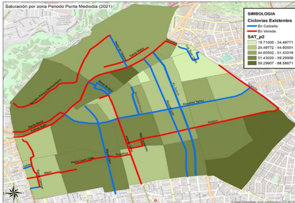
FIGURA Nº 5.2-100: SATURACION VERSUS CICLOVIAS SITUACION ACTUAL AÑO 2021
