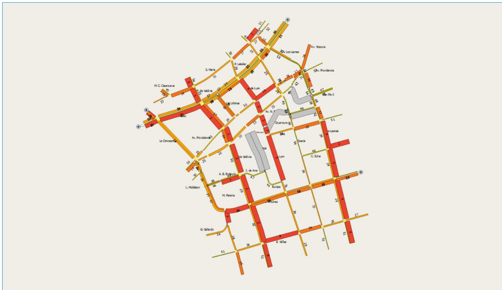
FIGURA N° 5.2-71: VELOCIDAD SIMULADA ÁREA DE MICROSIMULACIÓN 1 PLAN DE PROYECTOS PUNTA TARDE
