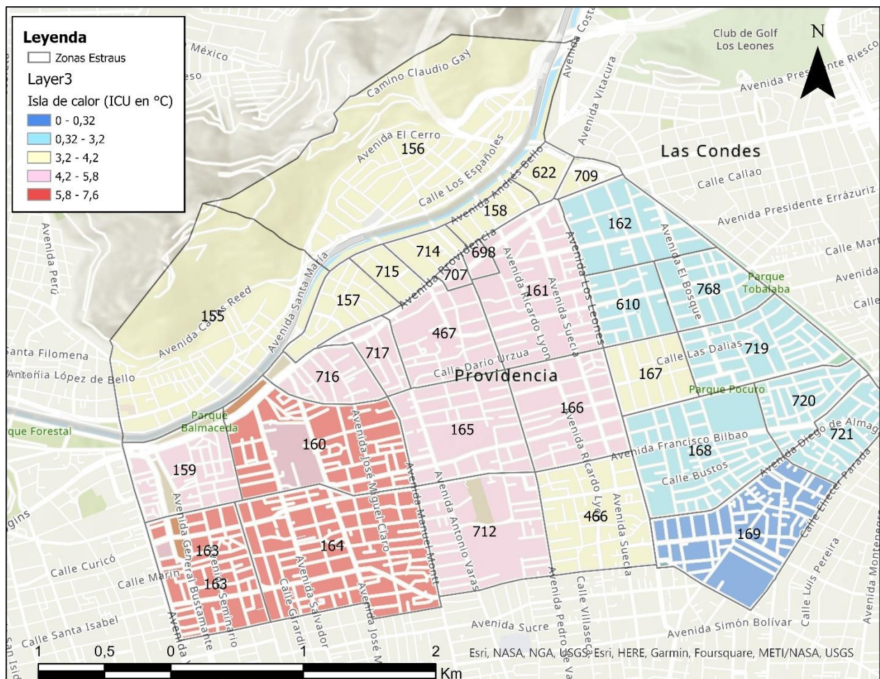
FIGURA Nº 4.1-37: VALOR PROMEDIO ICU DIURNA DE VERANO POR ZONA ESTRAS, PROVIDENCIA
