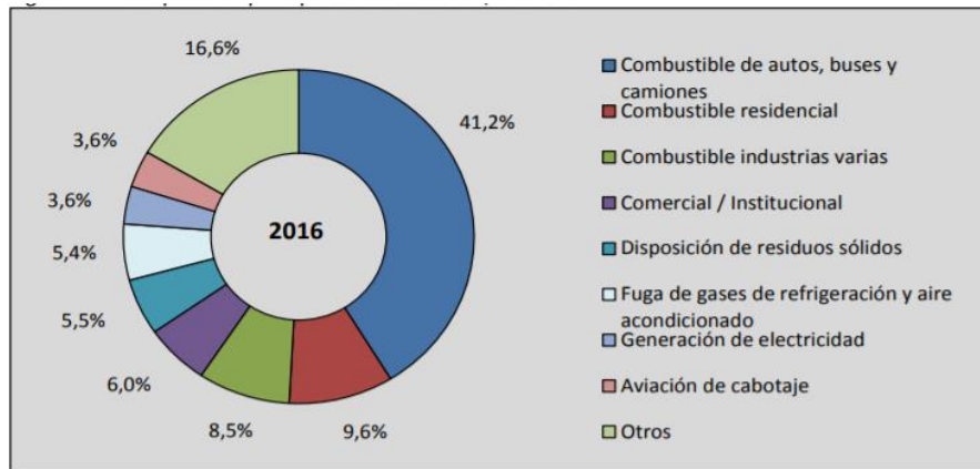
FIGURA N° 4.1-34: FUENTES DE EMISIÓN AL 2016 EN LA REGIÓN METROPOLITANA
