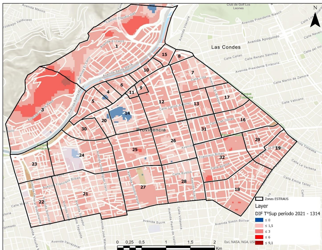
FIGURA N° 2.2-69: DIFERENCIA TEMPERATURA SUPERFICIAL VERANO 2013-14 Y VERANO 2020-21 PARA LA COMUNA DE PROVIDENCIA
