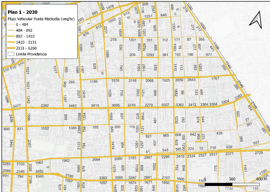
FIGURA Nº 4.8-59: FLUJO TOTAL SECTOR CENTRO CIVICO – PLAN 1 2030 PUNTA MEDIODÍA
