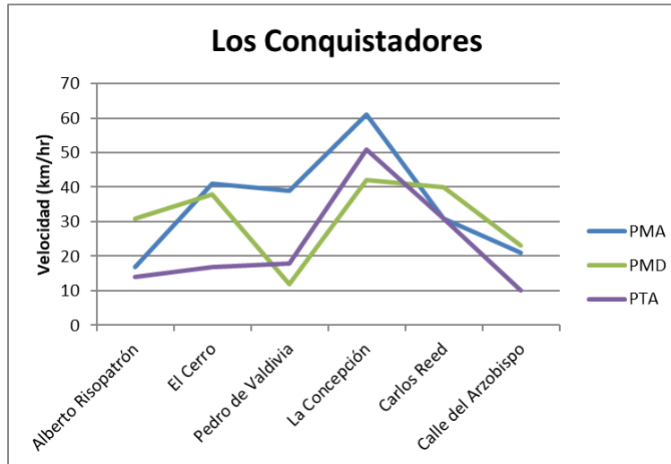
FIGURA Nº 3.1-30: PERFIL DE VELOCIDADES – LOS CONQUISTADORES / BELLAVISTA
