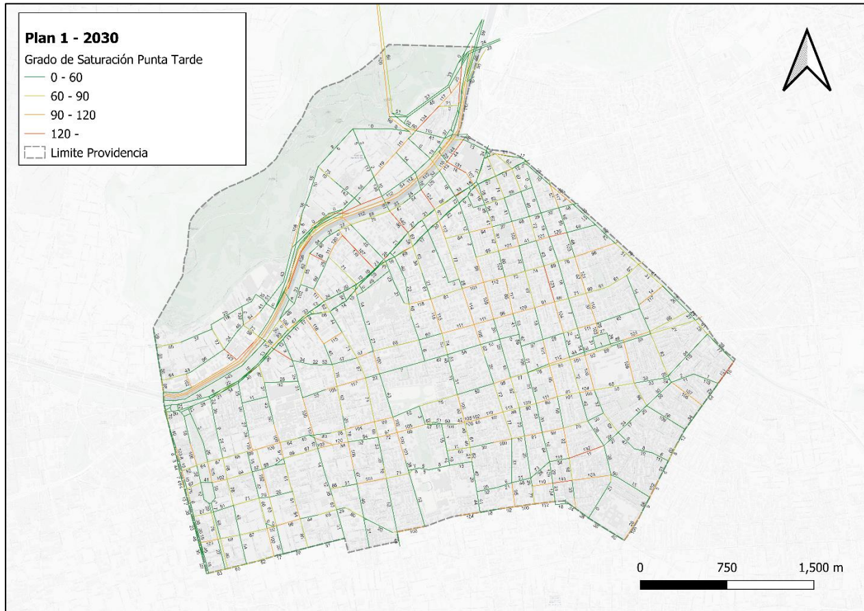
FIGURA Nº 4.8-62: GRADO DE SATURACIÓN DE LA RED – PLAN 1 2030 PUNTA TARDE
