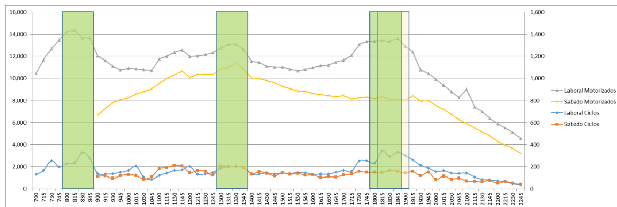
FIGURA Nº 2.3-31: COMPARACIÓN DE HISTOGRAMAS DE FLUJO Y PERIODIZACIÓN – DÍA LABORAL
