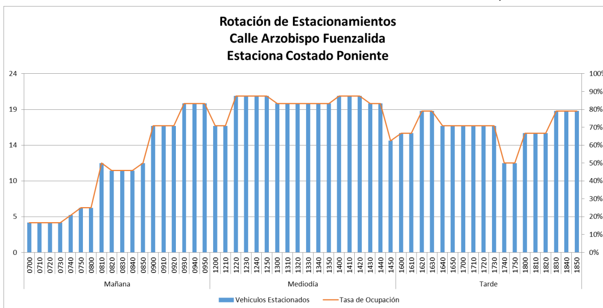
FIGURA Nº 3.1-15: PERFIL HORARIO DE VACANCIA Y OCUPACIÓN – CALLE ARZOBISPO FUENZALIDA, COSTADO PONIENTE
