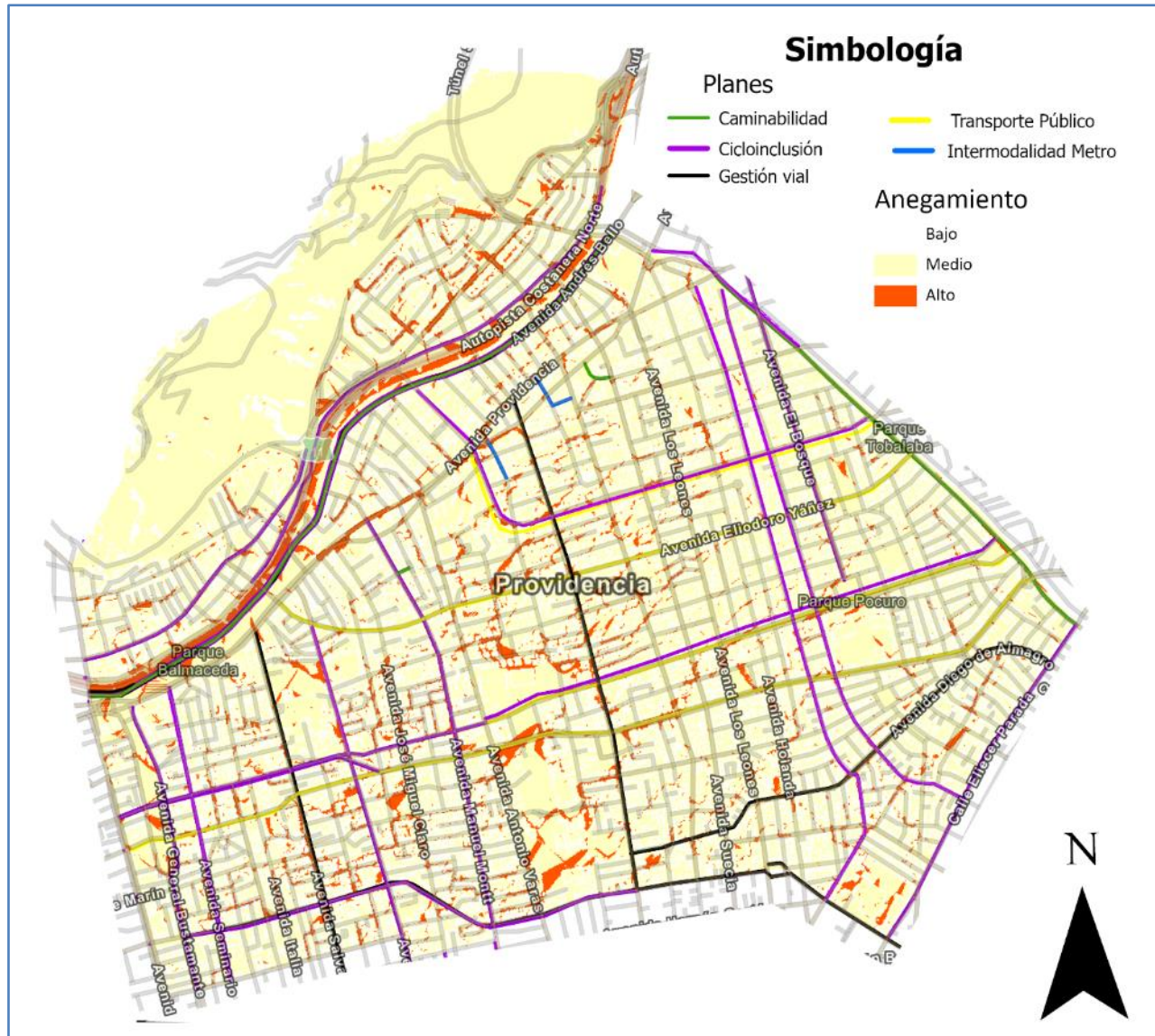
FIGURA Nº 5.2-108: ÁREAS DE ANEGAMIENTO ACTUAL Y PROYECTOS
