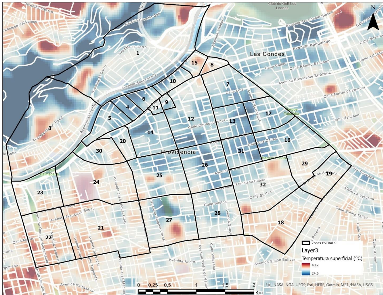
FIGURA N° 2.2-67: PROMEDIO TEMPERATURA SUPERFICIAL, VERANOS 2013-14 A 2020-21 PARA LA COMUNA DE PROVIDENCIA
