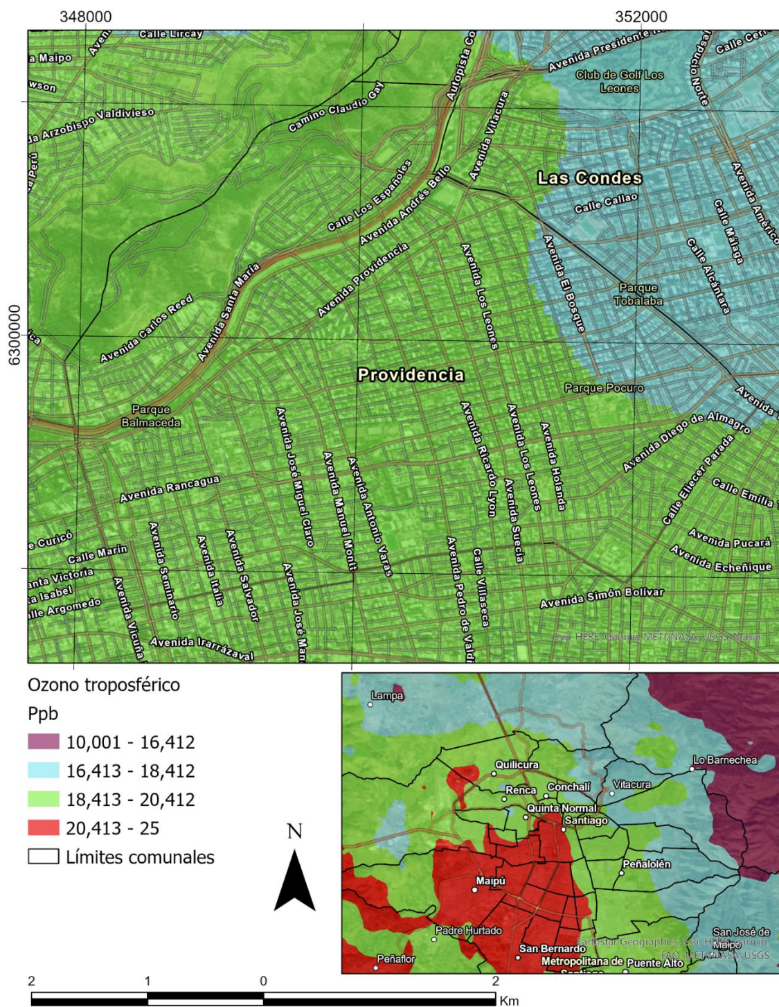
FIGURA Nº 2.2-82: DISTRIBUCIÓN ESPACIAL O3 EN VERANO PARA LA COMUNA DE PROVIDENCIA
