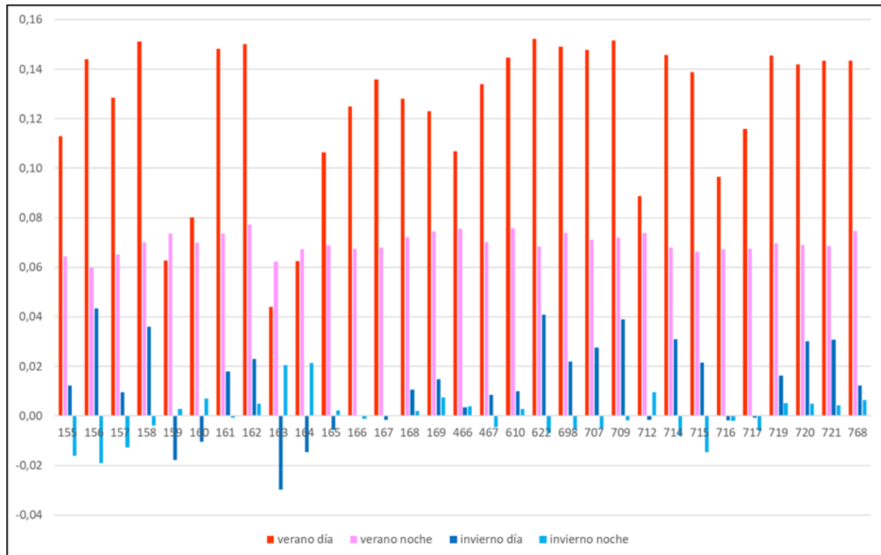
FIGURA N° 4.1-40: TENDENCIA TEMPERATURA DE SUPERFICIE (°C/AÑO) POR ZONA ESTRAS Y ESTACIÓN.
