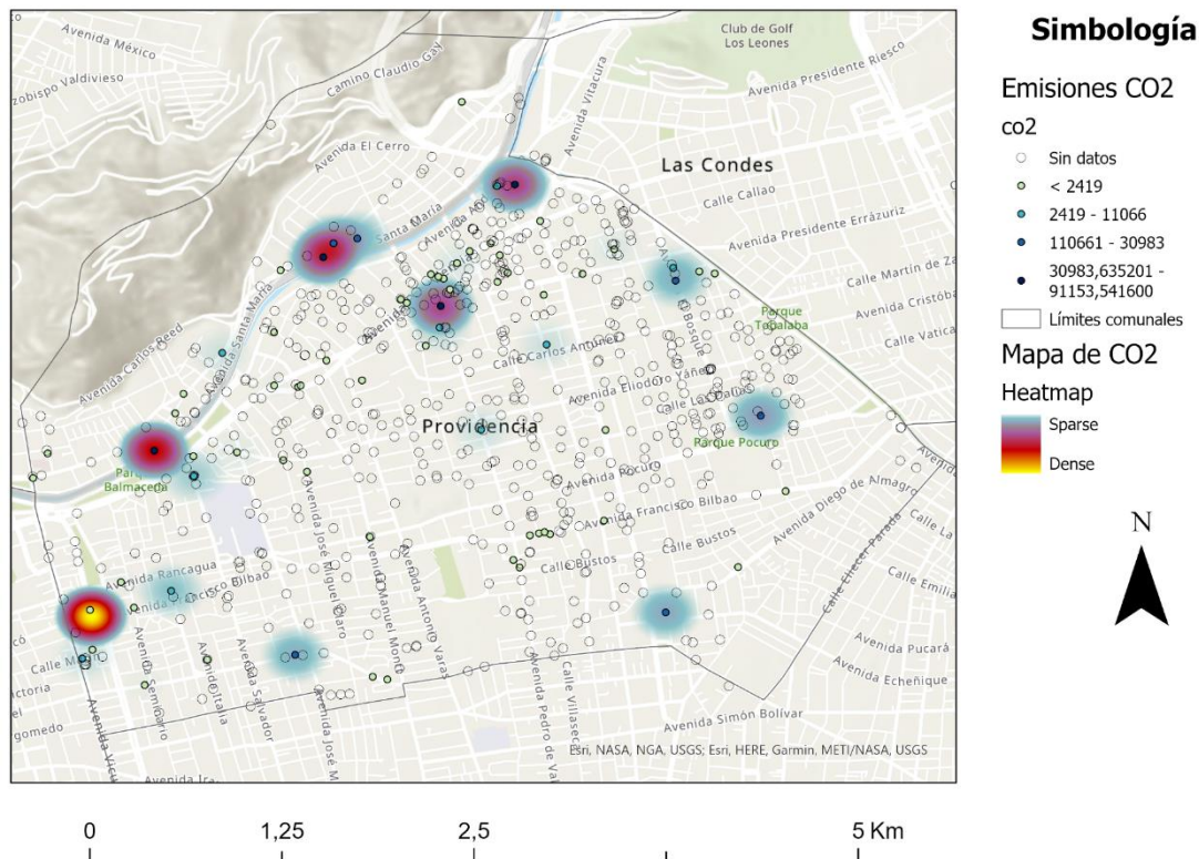
FIGURA Nº 2.2-88: EMISIONES EN PROVIDENCIA DE CO 2 (TONELADAS POR AÑO) AÑO 2016
