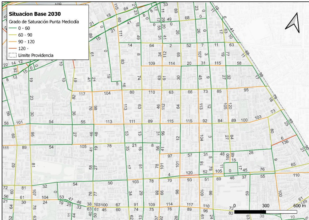
FIGURA Nº 4.8-24: GRADO DE SATURACIÓN SECTOR CENTRO CIVICO – SITUACIÓN BASE 2030 PUNTA MEDIODÍA
