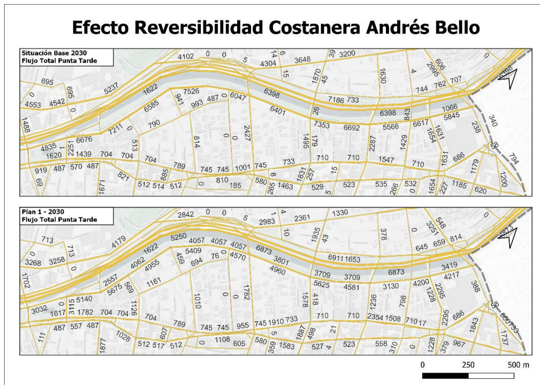
FIGURA N° 4.9-40: EFECTO DE LA REVERSIBILIDAD DE ANDRÉS BELLO – FLUJO TOTAL PUNTA TARDE 2030
