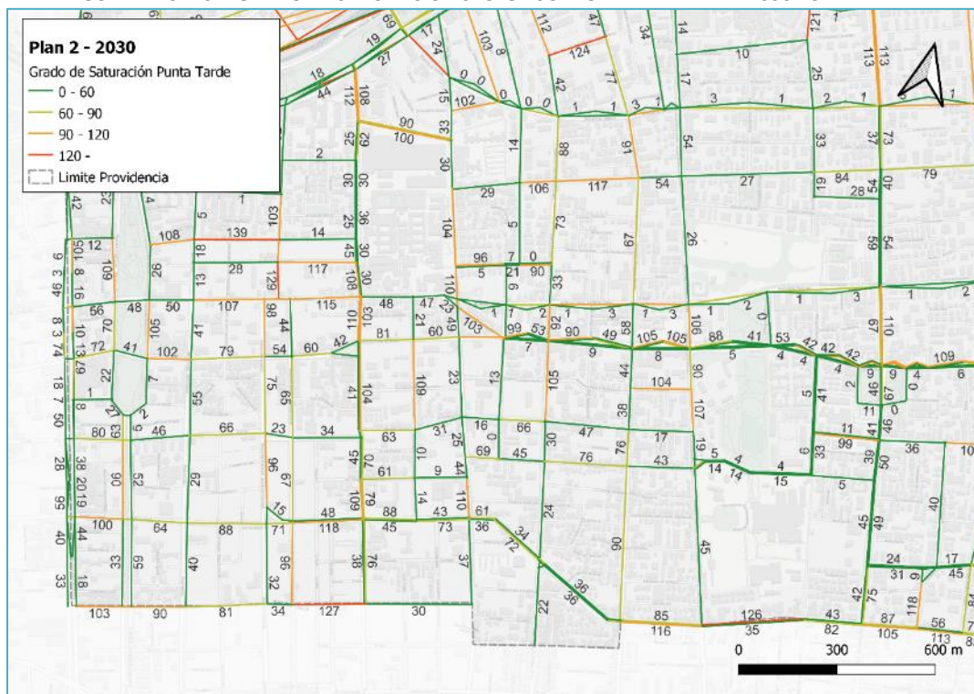
FIGURA Nº 5.2-34: GRADO DE SATURACIÓN SECTOR SURPONIENTE– PLAN 2 2030 PUNTA TARDE
