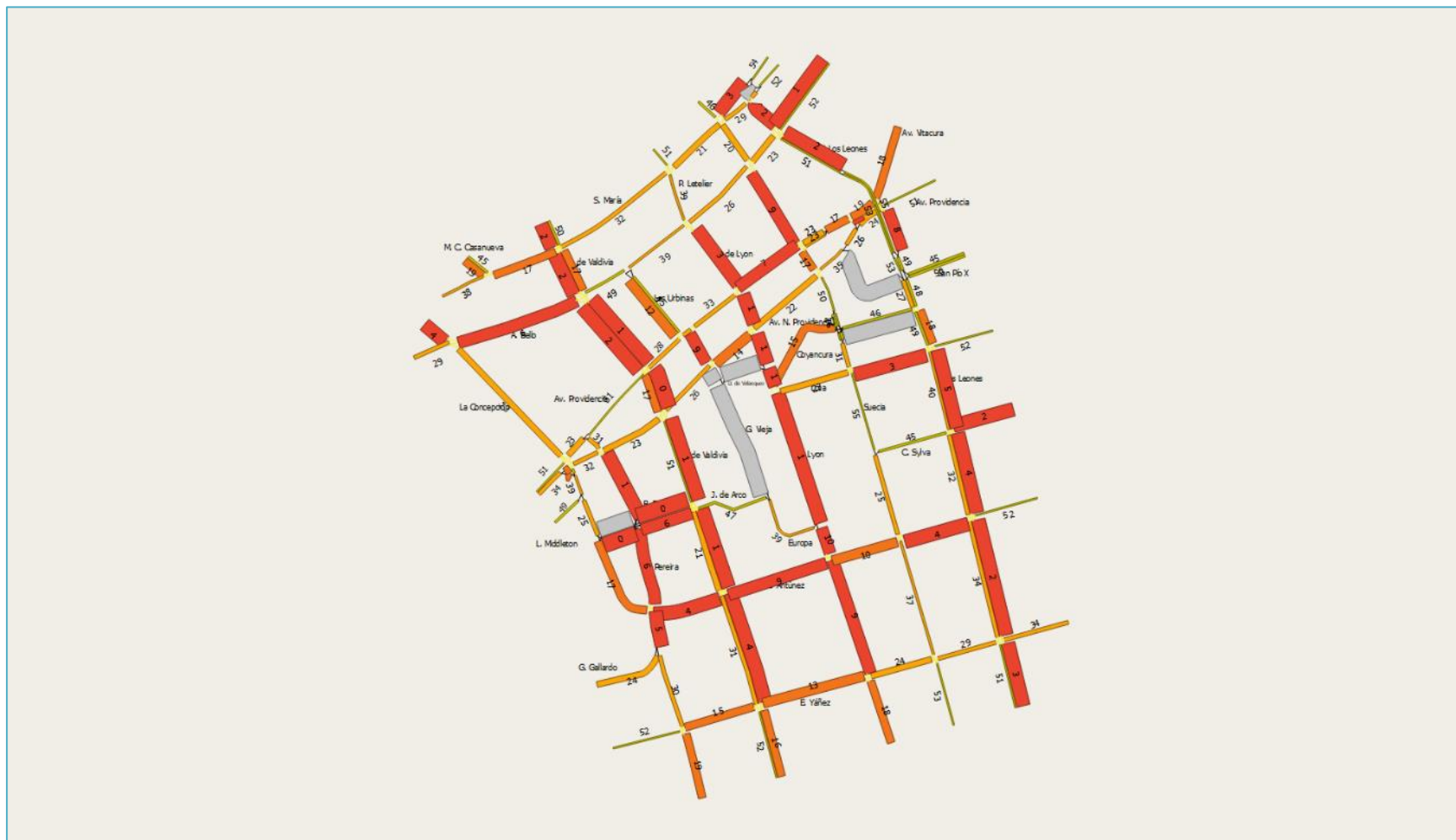
FIGURA Nº 5.2-51: VELOCIDAD SIMULADA ÁREA DE MICROSIMULACIÓN 1 SITUACIÓN BASE PUNTA TARDE
