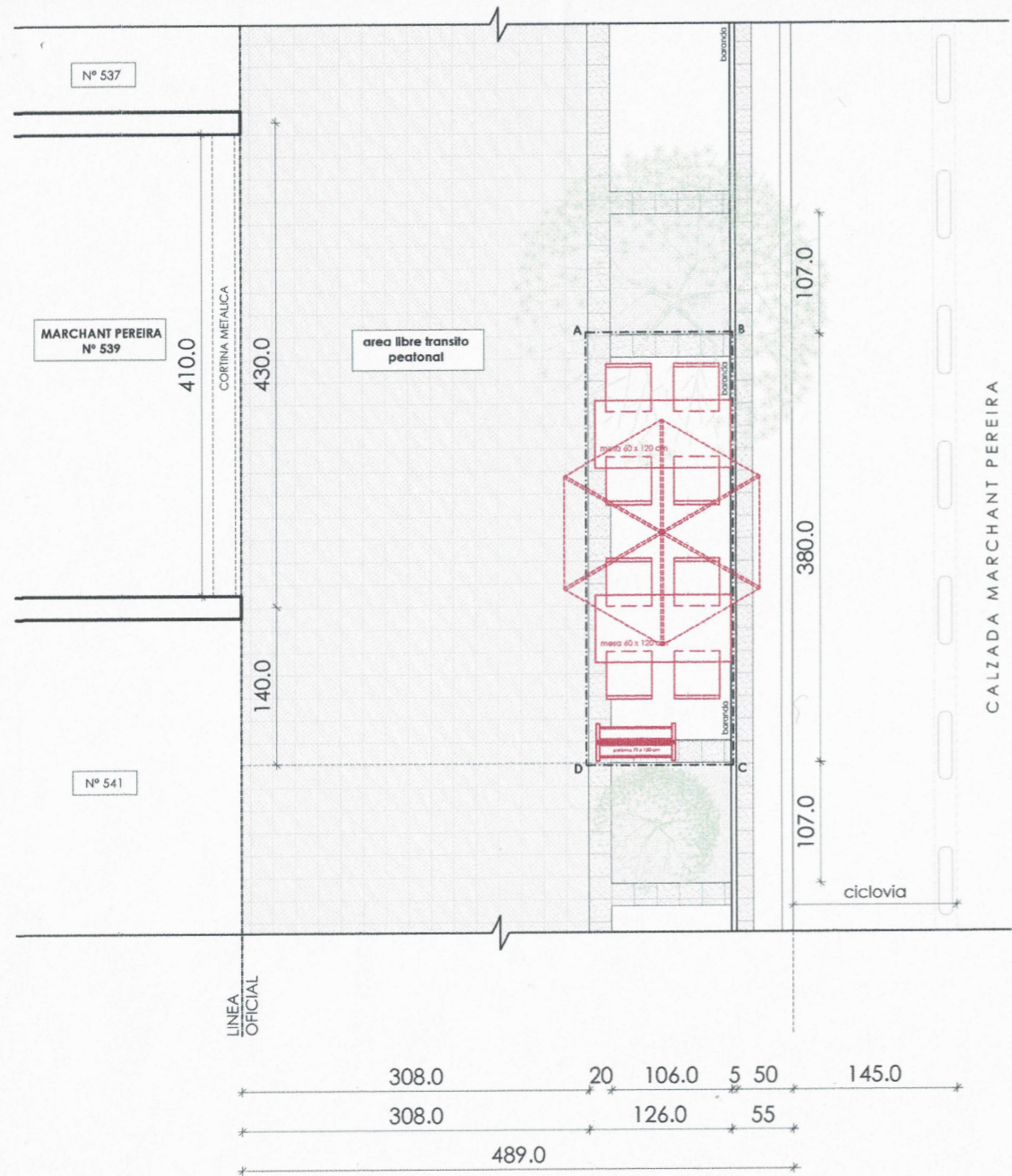
PLANTA
