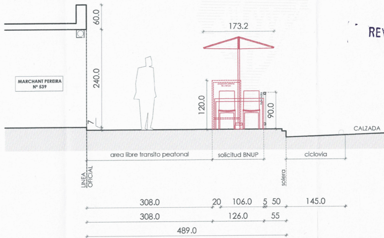
CORTE TRANSVERSAL
