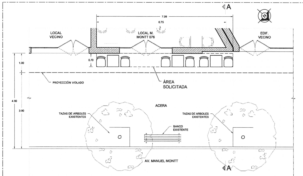
PLANTA DE ARQUITECTURA
