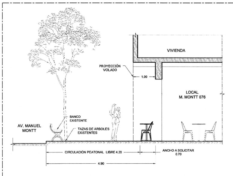
CORTE A
