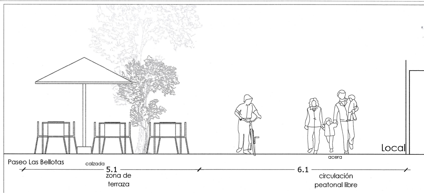
CORTE A-A'
