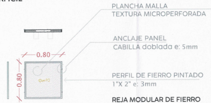
DETALLE SEPARADOR esc 1:50
