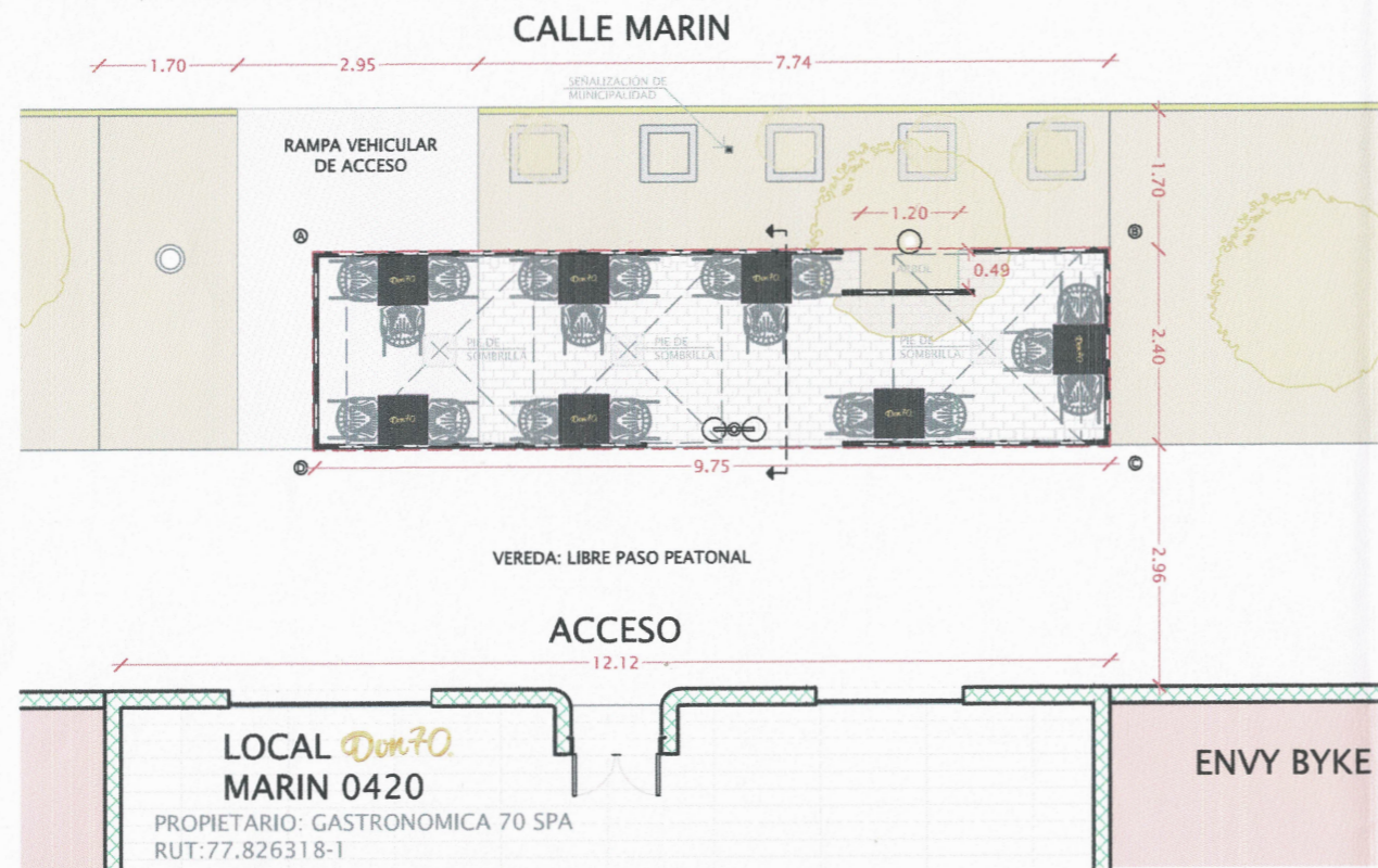
PLANTA GENERAL DE DISTRIBUCIÓN esc 1:100
