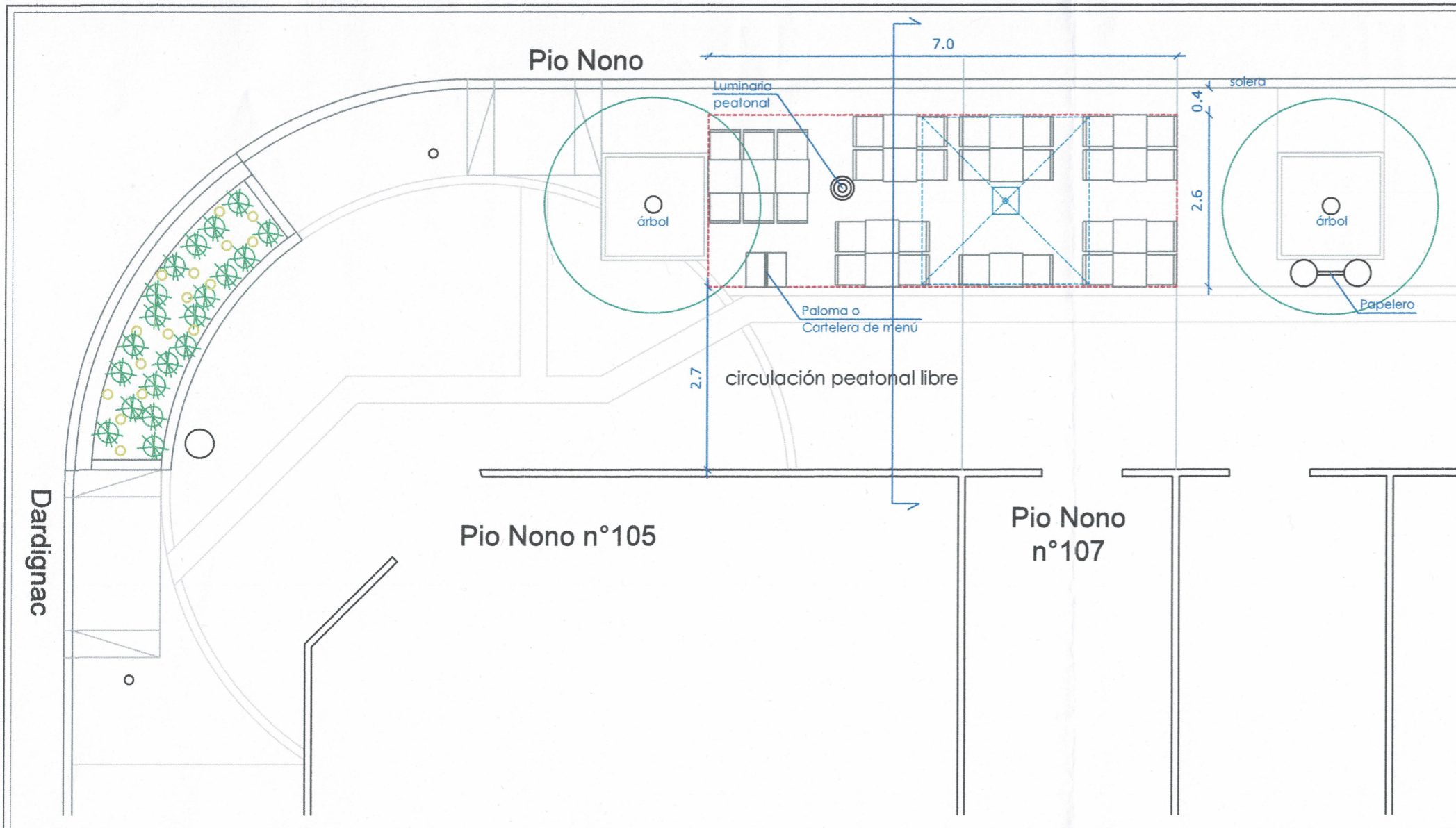
PLANTA
