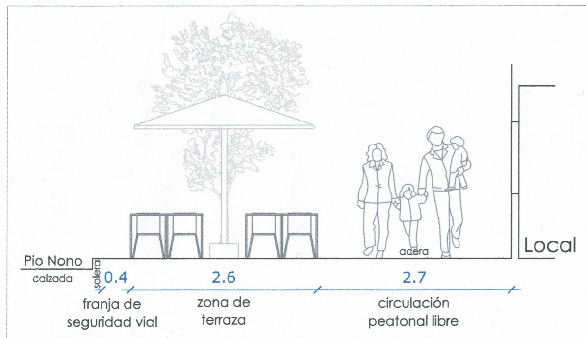
CORTE A-A'
