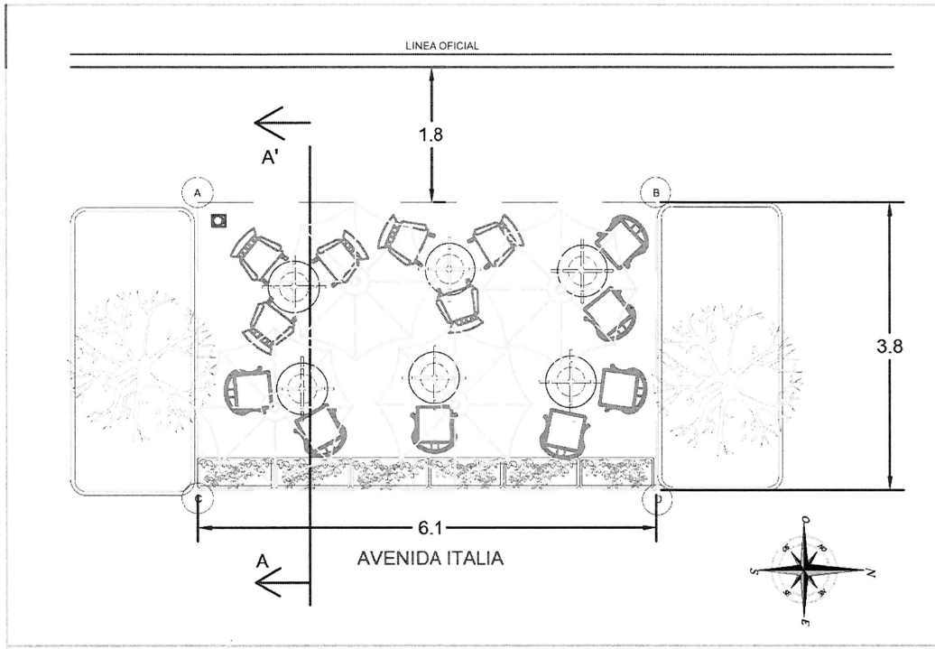
PLANTA 1:50
