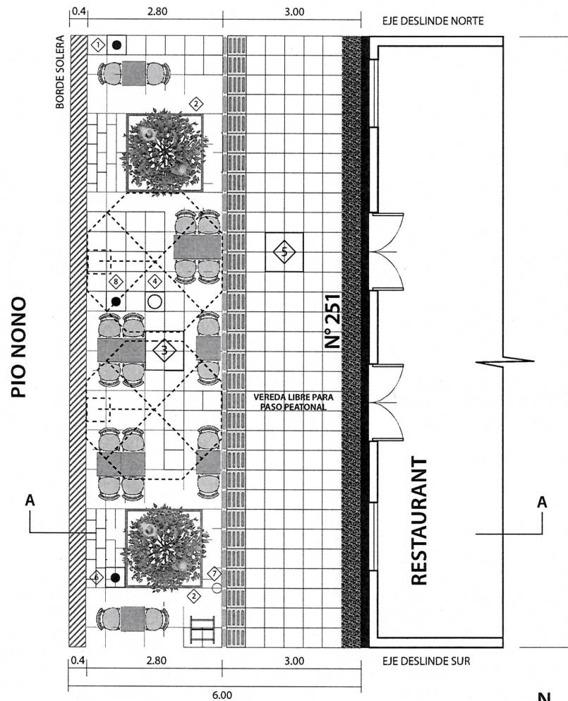
PLANTA SITUACIÓN PROPUESTA MOBILIARIO MESAS Esc. 1:75
