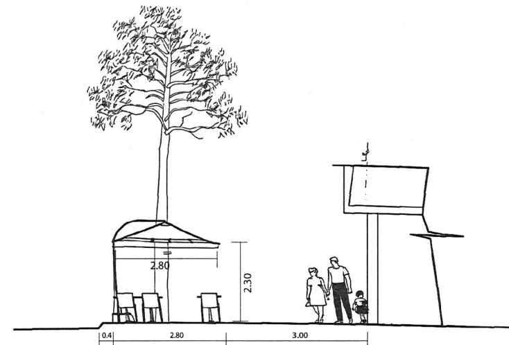
CORTE A - A_ Esc. 1:75
