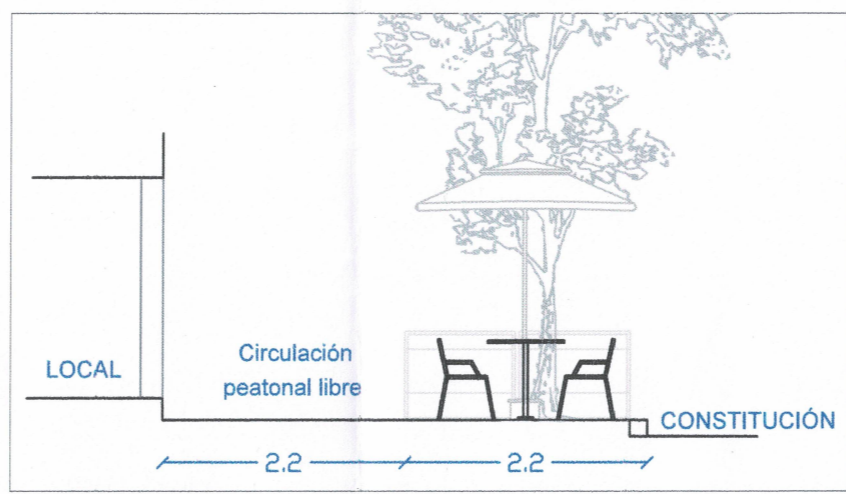
CORTE B-B'
