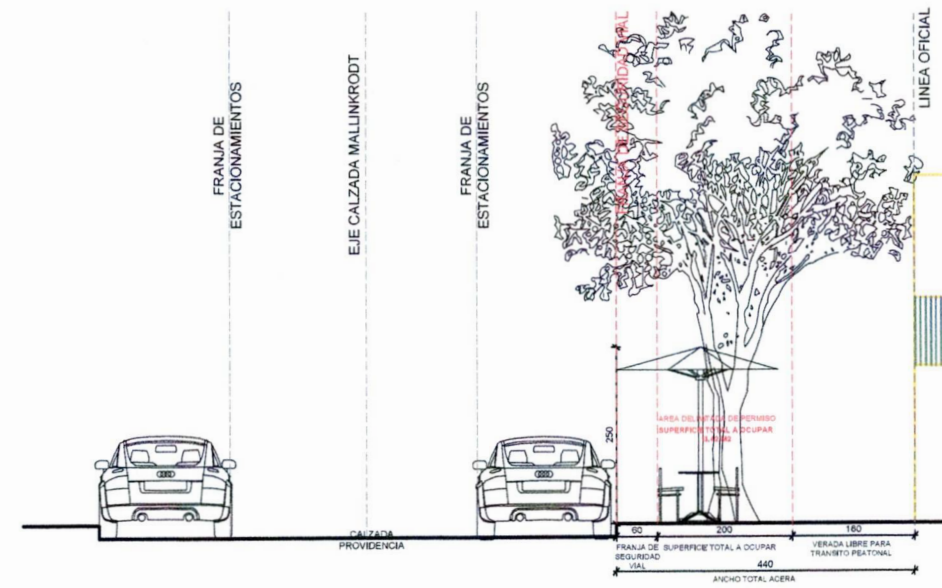
CORTE TRANSVERSAL A-A'
