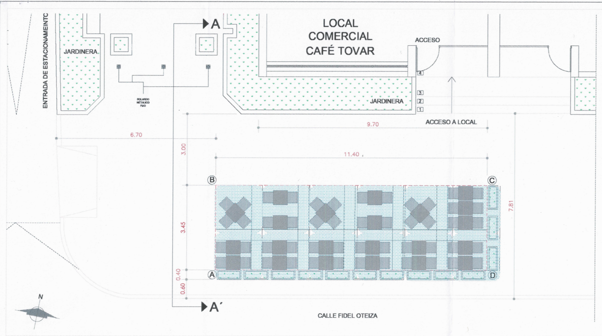
PLANTA DISTRIBUCIÓN
