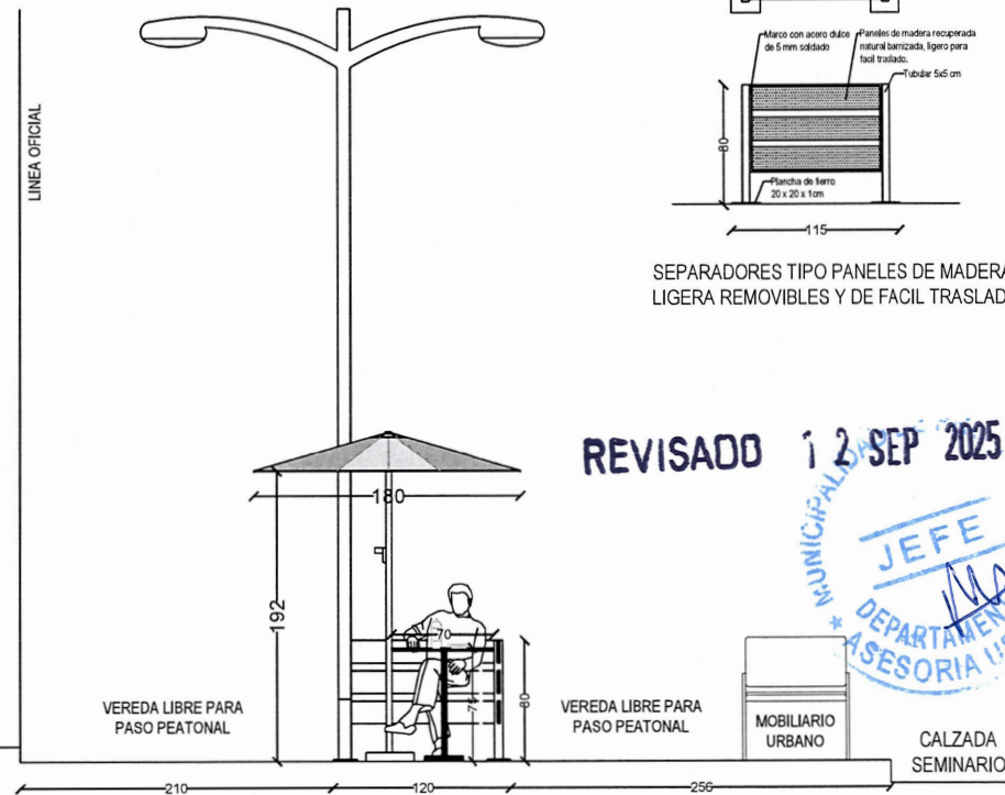
CORTE A-A
