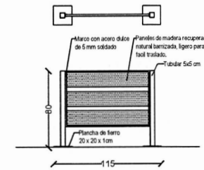
SEPARADORES TIPO PANELES DE MADERA LIGERA REMOVIBLES Y DE FÁCIL TRASLADO.
